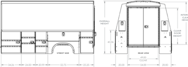
108” CA DRW
