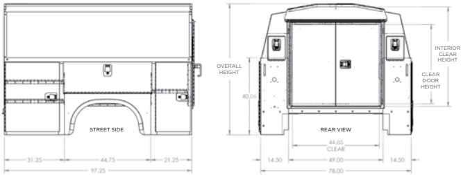
56” CA SRW
