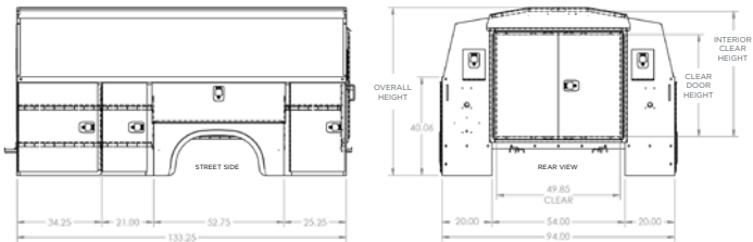
84” CA DRW
