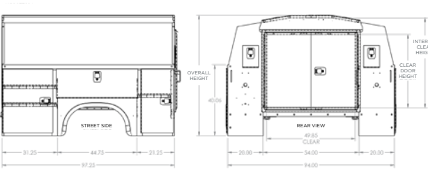
56” CA DRW
