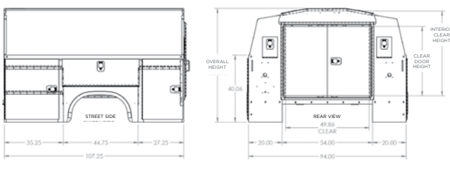
60” CA DRW
