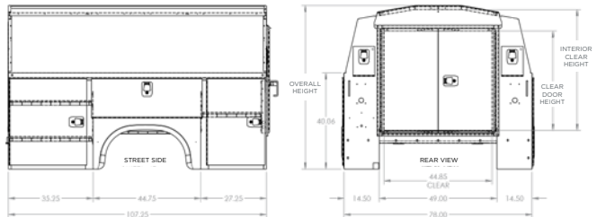
60” CA SRW
